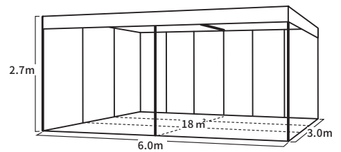
2小間 立面図
